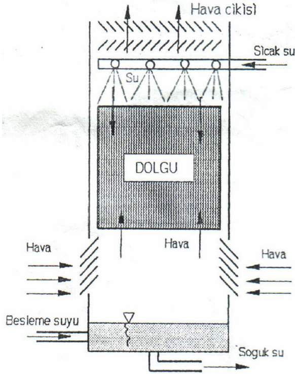
Şekil 1. Soğutma kulesi, [3]
