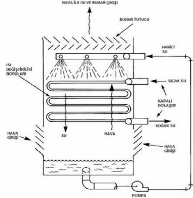
Şekil 4. Kapalı tip soğutma kulesi, [1]
