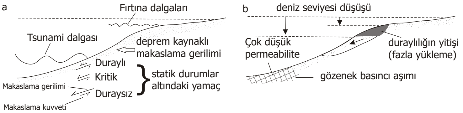
Şekil 3. Denizde yamaç kaymalarındaki yaygın mekanizmalar (Einsele vd., 1996'dan değiştirilerek)
