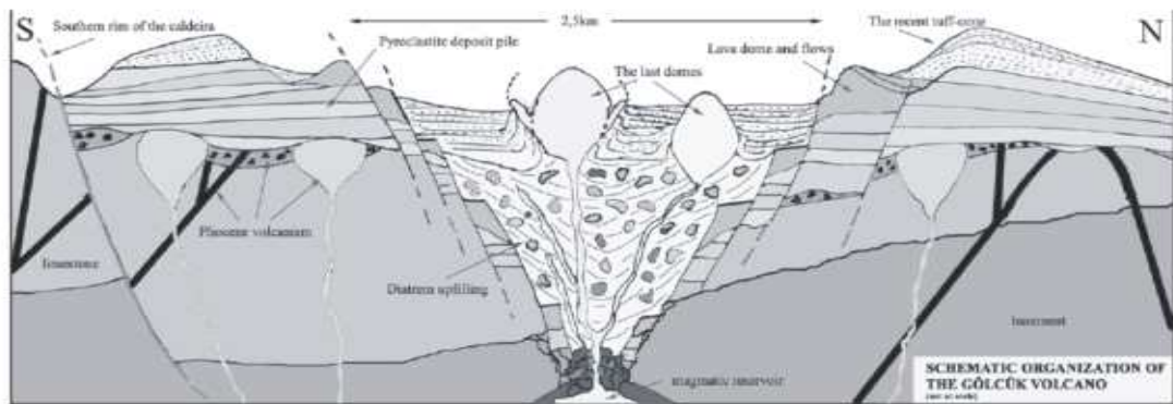
Şekil 2. Gölcük volkanı ve yakın çevresinin jeolojisi (a), Gölcük çevresinden geçen jeolojik enine kesit (b) (Platevoet ve diğ. 2008'den alınmıştır.)
